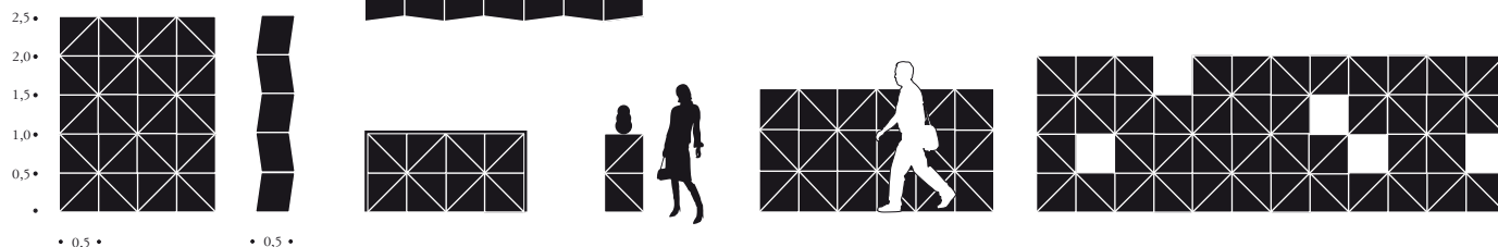
Konfigurationsbeispiele: Länge beliebig, Höhe max. 5 Elemente ohne Abstützung, Öffnungen möglich
